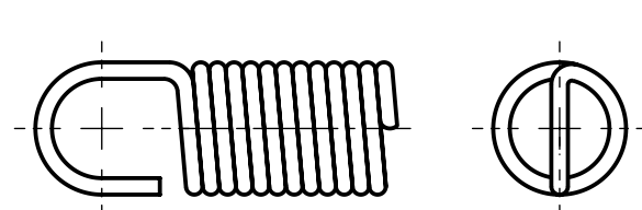
Hákové oko
