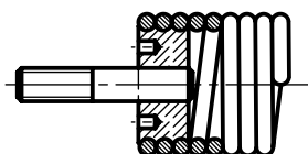
Zátka se závitem - počet zašroubovaných závitů 2 - 4
