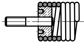
Bouchon fileté - 2 à 4 spires vissées
